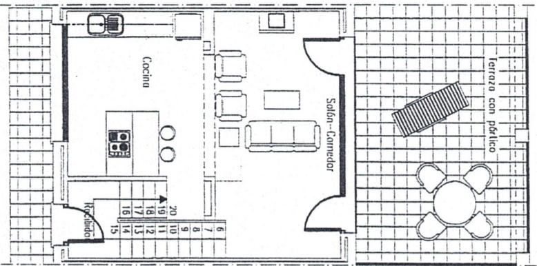
PLANTA ACCESO
